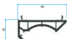
АДАПТОР ТРЪБА 63100
