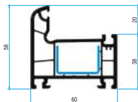
КАСА 63020
