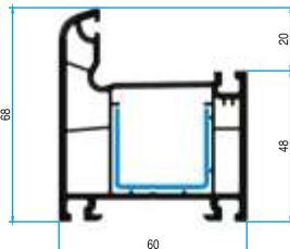
КАСА 63030
