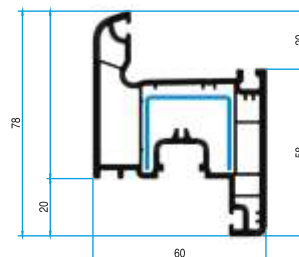
КРИЛО ПРОЗОРЕЦ 63040
