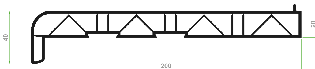
ПОДПРОЗОРЕЧНА ДЪСКА 63200
